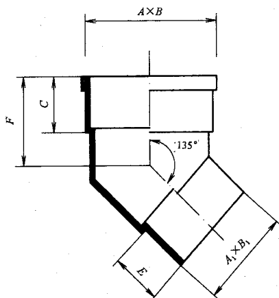
图 A1 矩形管 135° 弯管
