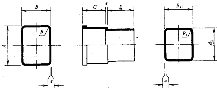
图3 矩形管件承口、插口及壁厚
