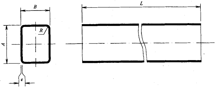
图1 矩形管材外形尺寸与壁厚
